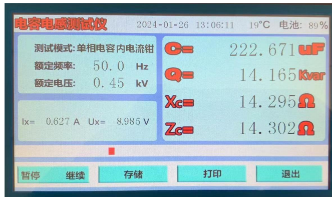
单相电容测试界面 图四
